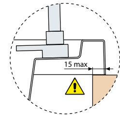
DETALLE DE BAÑERA EMPOTRADA
