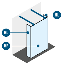
KUADRA HF KUADRA HL x2 STABILISATIONSSTANGE (im Lieferumfang)
