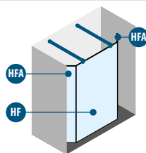
KUADRA HF KUADRA HFA x2 STABILISATIONSSTANGE (im Lieferumfang)
