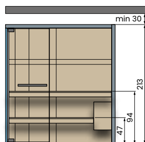
ANGLE À DROITE
