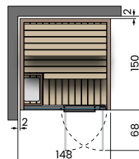
ANGLE À GAUCHE
