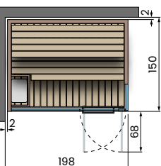
ANGLE À GAUCHE
