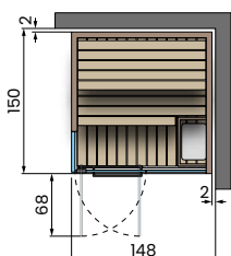
ANGLE À DROITE
