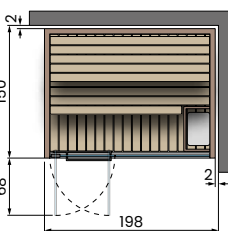
ANGLE À DROITE
