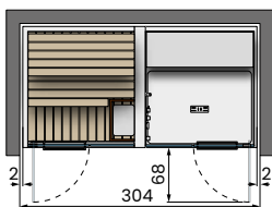
EN NICHE W
