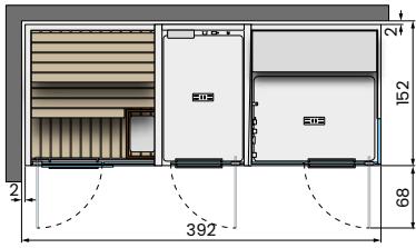
CENTRE DE MUR G
