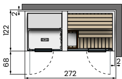
ANGLE À DROITE
