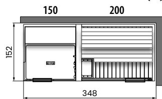
ANGLE À DROITE - VERRE (G)
