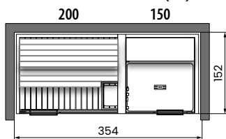
EN NICHE - BOIS (W)
