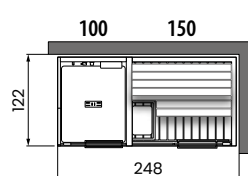
ANGLE À DROITE
