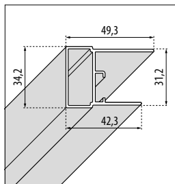
Verbreiterungsprofil als Ersatz des standard Profils +15mm
