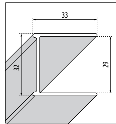
MUURPROFIEL / PROFILÉ MURAL VOOR / POUR OPERA FH
