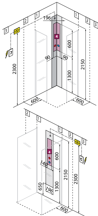
Regendouche / Douche zénithale 200x200 mm
