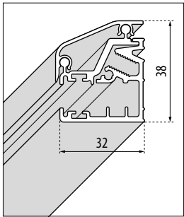
WALL for GALA A / G / 1B / 2P / 2A / R
