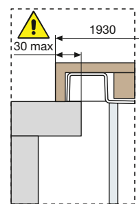
Detalhe para caso de instalação de embutir
