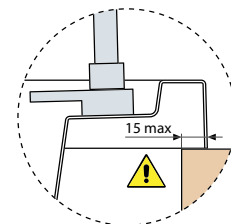
Detalhe para caso de instalação de embutir
