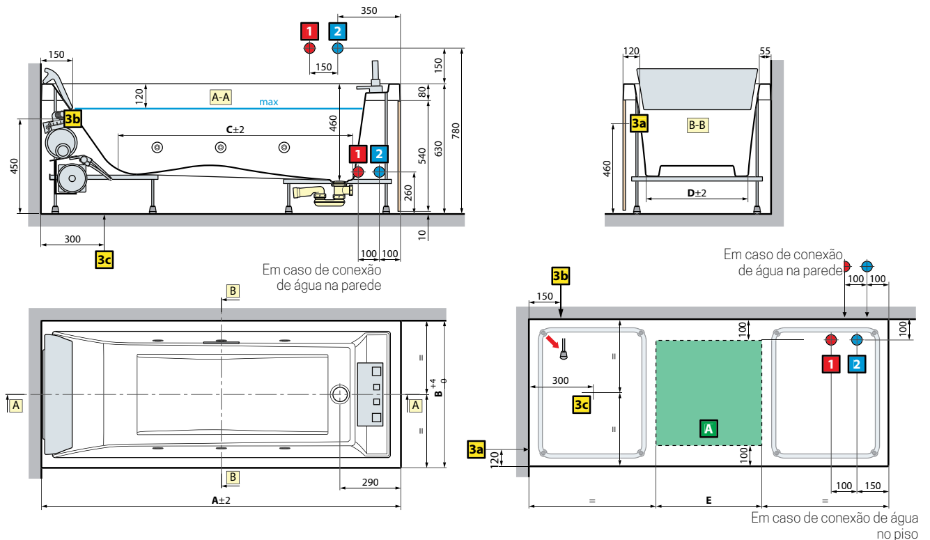
Detalhe para caso de instalação de embutir
