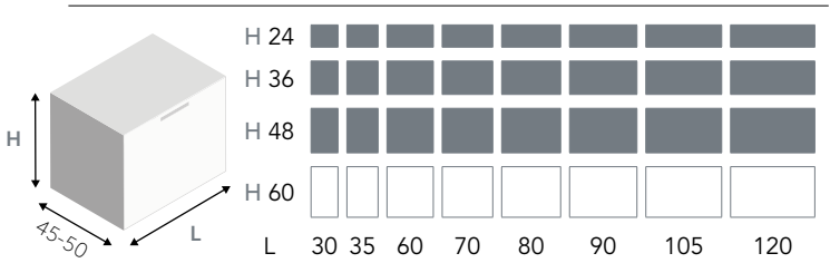
1 TIROIR
